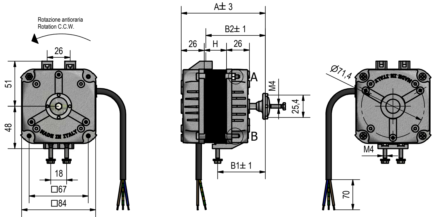
Versione con dado Version with nut
