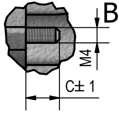
Versione senza dado Version without nut
